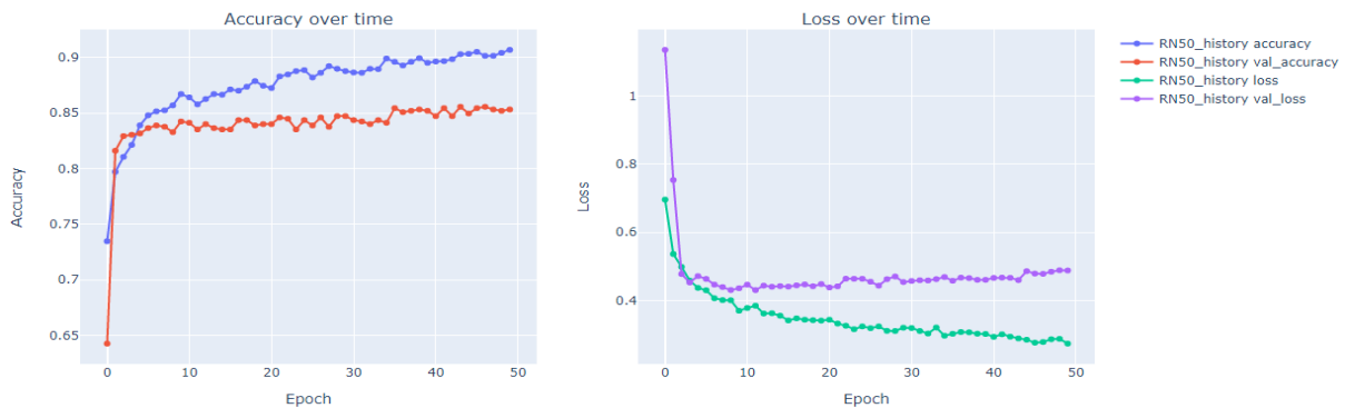
Şekil 4. ResNet50 modelinin eğitim başarımları ve kayıpları için grafiksel gösterimi.
