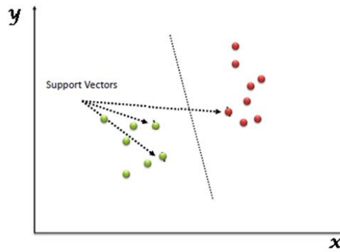
Şekil 4. Destek vektör makineleri sınıflandırma örneği
