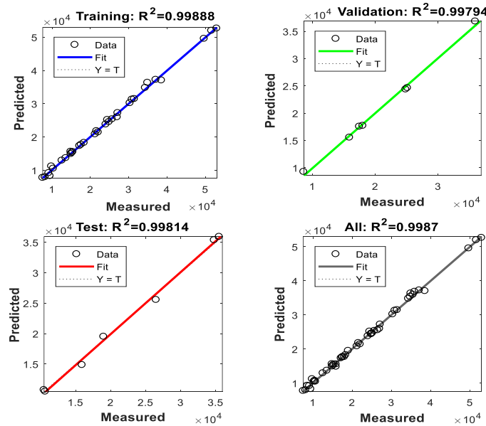
Şekil 8. Deneyisel değerler ile tahmin edilen değerler arasındaki ilişkiyi gösteren grafikler
