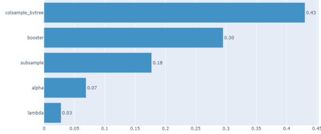
Şekil 2. TPE amaç fonksiyonuna göre sonucu en çok etkileyen parametreler.
