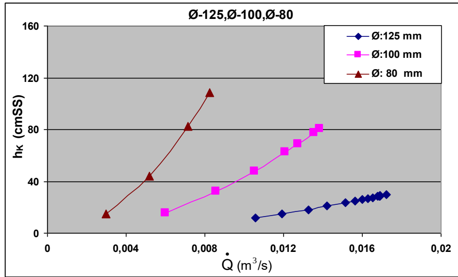
Şekil 6. Yük kayıp katsayısı ( h_k ) ve Akışkan debisine ( \dot{Q} ) ait deney sonuçları
