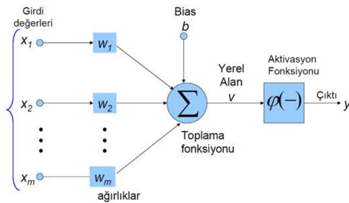
Şekil 3. Bir nörona ait blok diyagram modeli [10]
