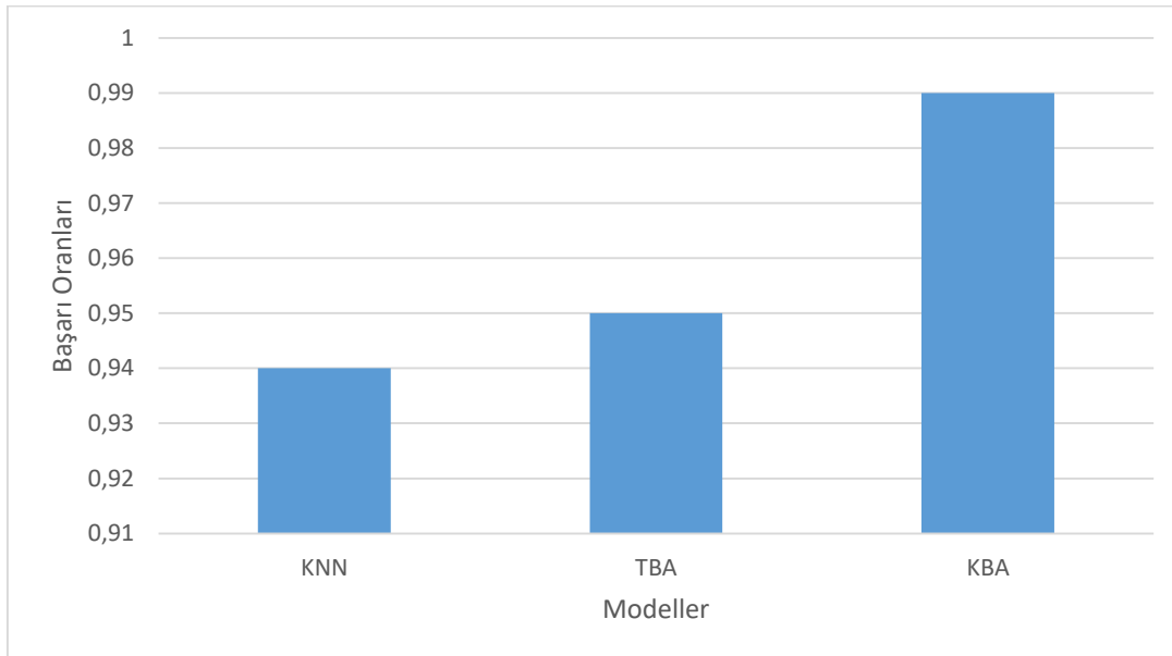
Şekil 1. Makine öğrenmesi modellerinin başarı oranları
