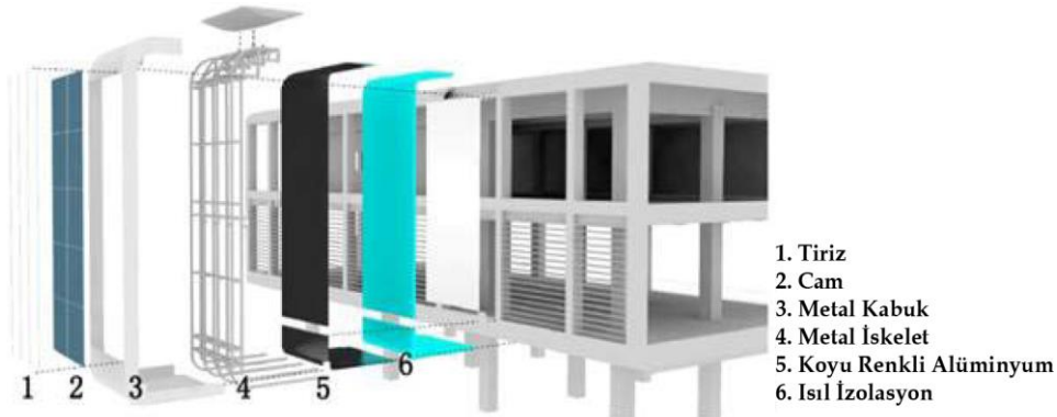
Şekil 10. P+ Binası ve binada kullanılan güneş bacasının katmanları ve kurgusu (Zha ve ark, 2017)
