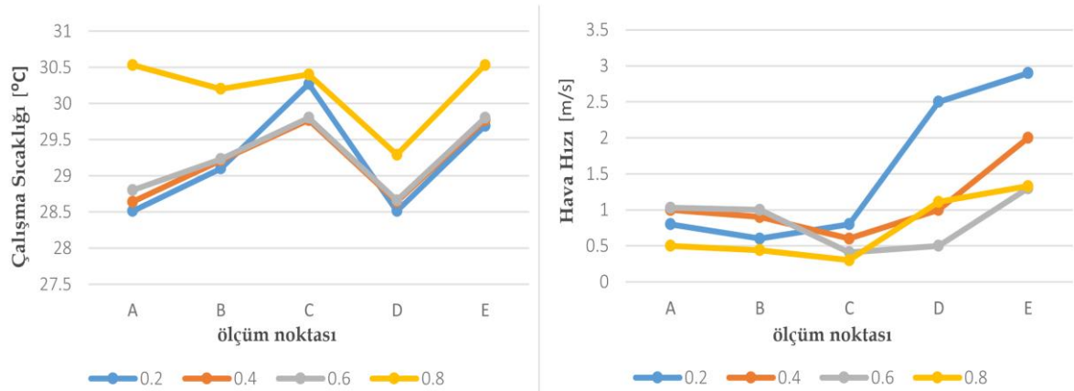
Şekil 13. İskenderiye'de Konut Binasının sıcaklık ve hava hızı ölçüm sonuçları (Mekawi ve Elgendy, 2016)
