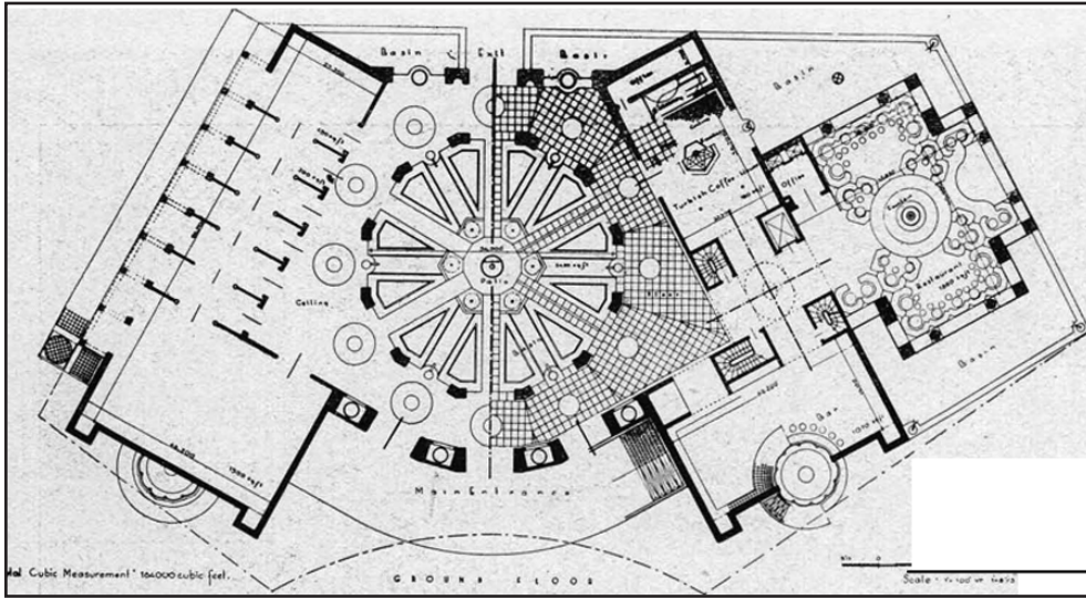
EK 5.a. Türk Sitesi'nin Zemin Kat Planı
