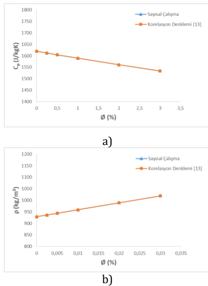
Şekil 4. Nanoakışkanın temel özelliklerin konsantrasyon oranına göre değişimi, a) Özgül ısı kapasitesi, b) Yoğunluk.
