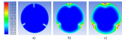
Şekil 5. Model 2 ve konsantrasyon oranı %3 olduğunda, boru eksen boyu farklı konumlarda ki kesitler için sıcaklık dağılımı a) 0,02 m, b) 1 m, c) 1,8 m.
