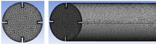
Şekil 2. Model 3'ün Ağ Yapısı.
