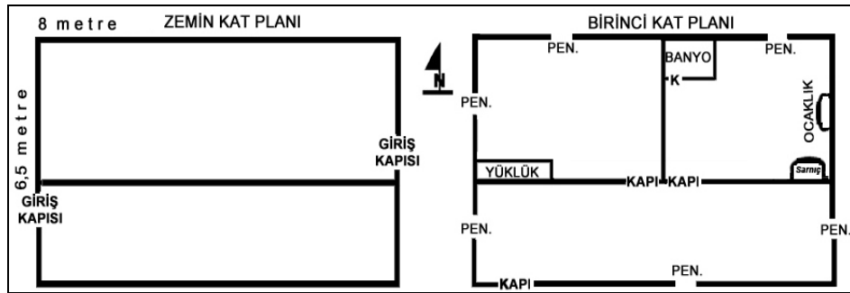
Şekil: 3- Kayaköy Taş Meskenlerinden En Yaygın Olan Plan Örneği
