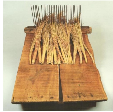
Fotoğraf 141: Süpürge otu tarama aracı
