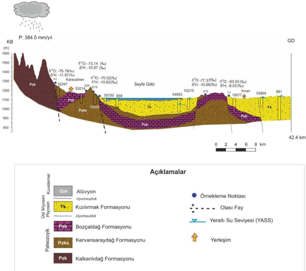
Şekil 8. Havzanın KB-GD hattında şematik izotopik değişim (Schematic representation of the change in stable isotope contents from NW to SE of the basin)
