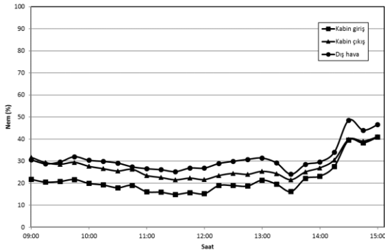
Şekil 18. Sistem üzerinde farklı noktalarda ölçülen rölatif nemlerin zamanla değişimi
