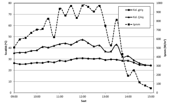
Şekil 19. Kolektör giriş-çıkışında ölçülen sıcaklıkların ve ışıınının zamanla değişimi
