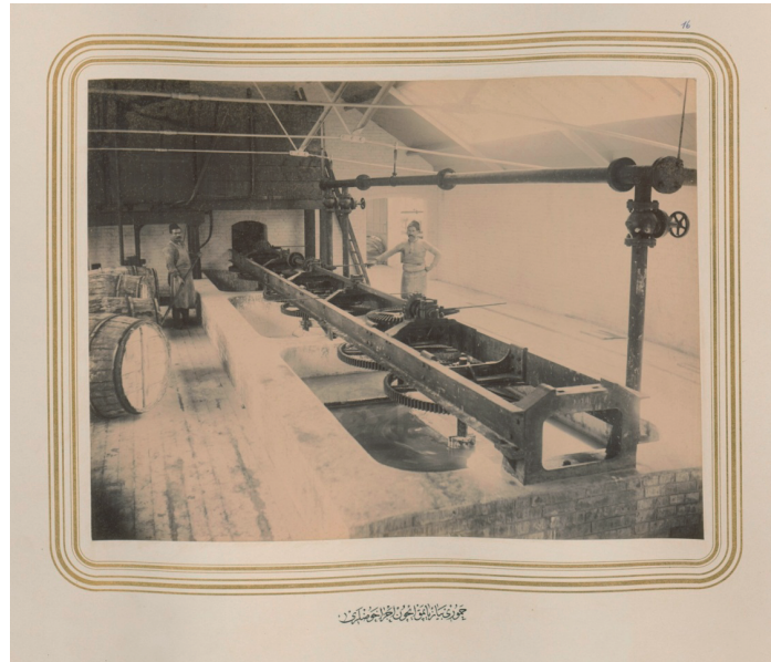
Fotoğraf 6: Kâğıdı Beyazlatmak İçin Kullanılan Kimyevi Madde Havuzları
