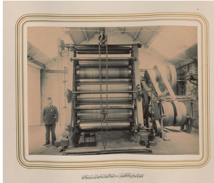
Fotoğraf 10: Kâğıtlara Cila Vermek İçin Kullanılan 40 Tonluk Sıcak Pres
