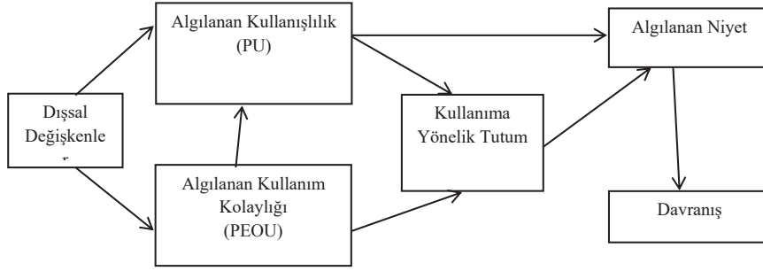
Şekil 1. TAM Modeli
