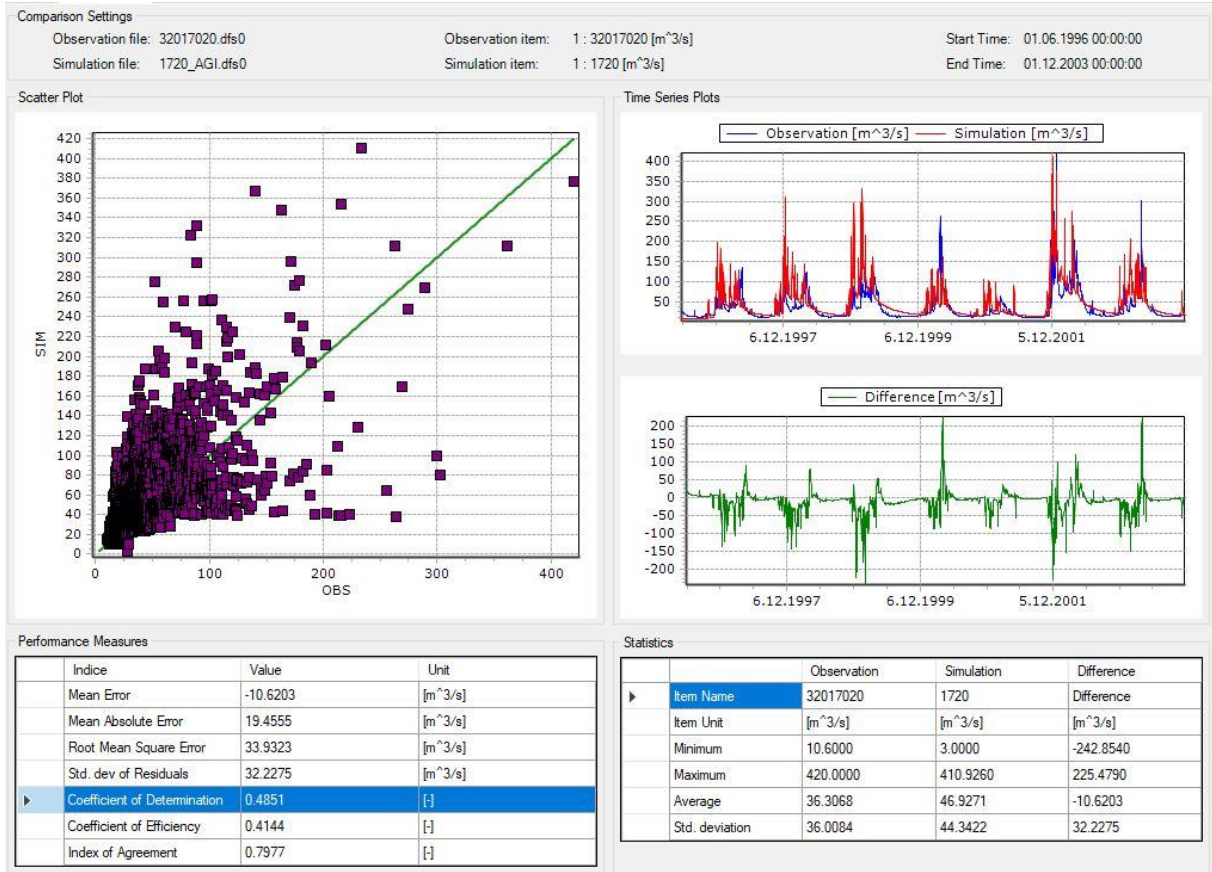
Şekil 7. 2 Numaralı alt havzada Göksu Nehri model sonuçları ile 1720 no'lu akım gözlem istasyonu akım değerlerinin karşılaştırılması
