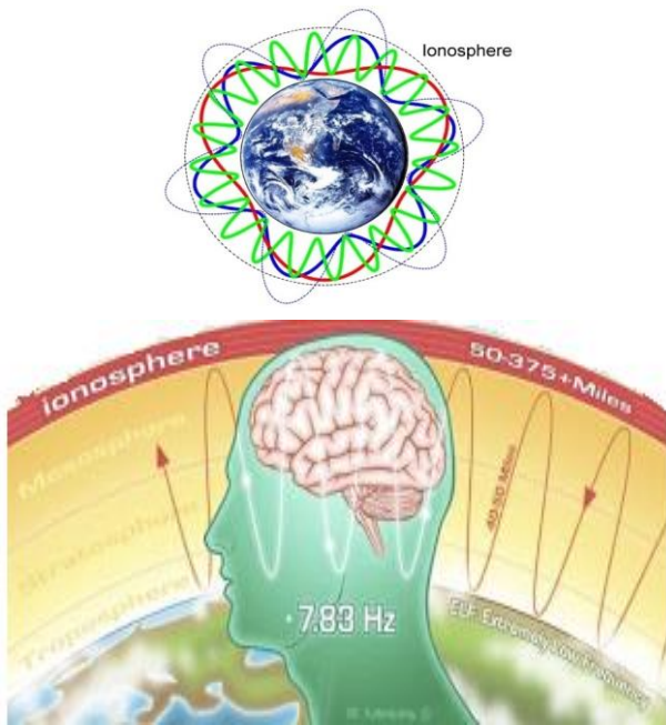
Şekil 5: Schumann rezonansı.
