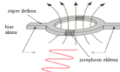
Şekil 2: Josephson eklemi.
