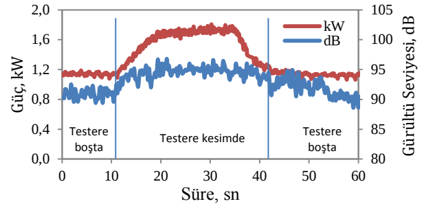
Şekil 2: Kesme işleminde zamana bağlı olarak oluşan güç ve gürültü seviyesi değerleri.
