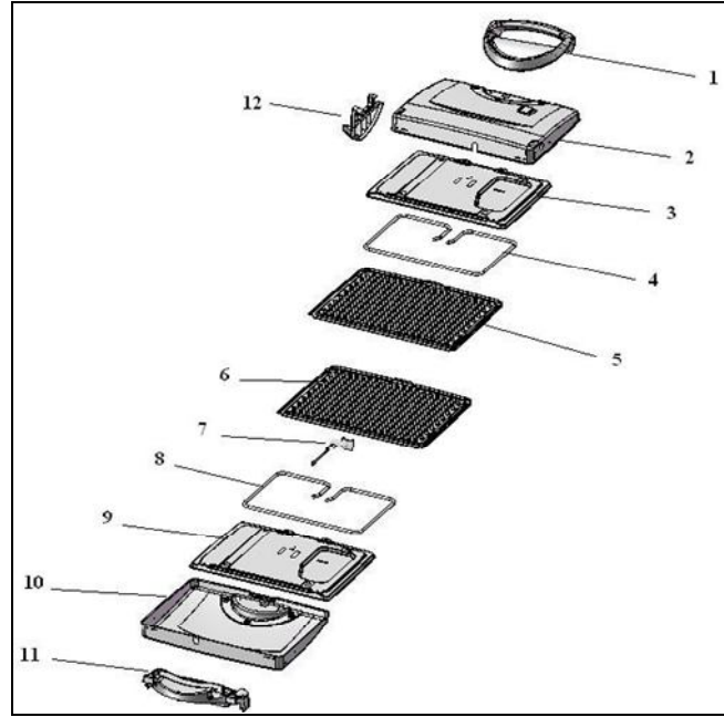
1. Üst kol; 2. Üst kapak; 3. Üst Galvaniz; 4. Üst Rezistans; 5. Üst Izgara; 6. Alt Izgara; 7. Termostat; 8. Alt Rezistans; 9. Alt Galvaniz; 10. Alt Kapak; 11. Alt Kol; 12. Menteşe.
