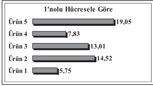
Şekil 11. 1'nolu hücresele yerleşim göre taşımada geçen süre yüzdeleri.
