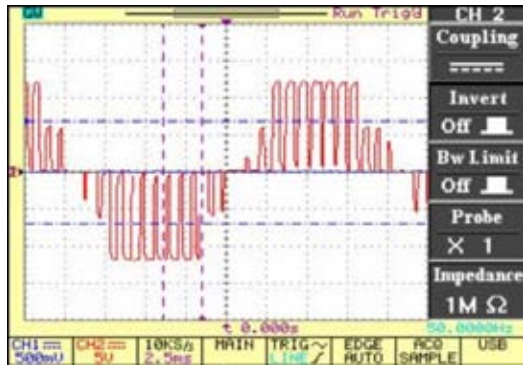
Şekil 10. Çok seviyeli eviricinin açık devre filtersiz çıkış voltajı (1/22 prob zayıflatması ile). Şekil 2’deki filtre devresi girişinden elde edilmiştir.
