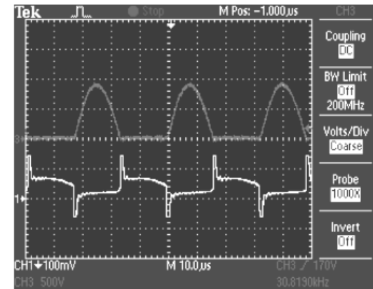
Şekil 6. BJT anahtarlama dalga şekilleri a) L vrb =15mH için b) L vrb =2mH için. (CH1:100mA/div, CH3:250V/div).
