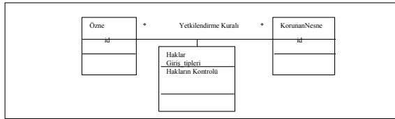
Şekil 2. Yetkilendirme şablonu (Euardo, 2001)
