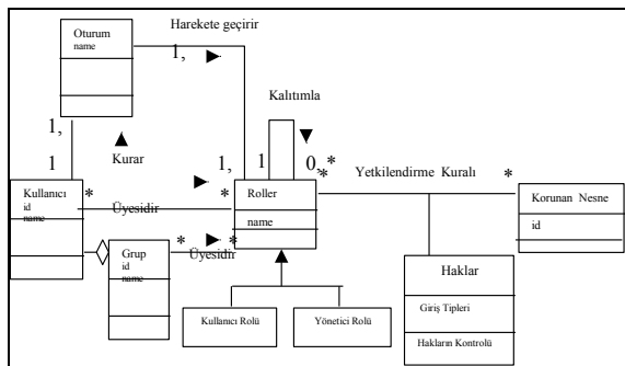
Şekil 3. Rollere göre giriş kontrol şablonu 5
