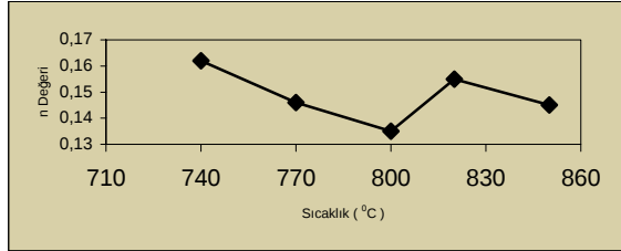
Şekil 3. SAE 1005 sac numunelerinin işlem sıcaklığı - n değeri değişimi
