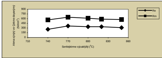
Şekil 1. SAE 1005 sac numunelerinin hadde yönünde, işlem sıcaklığı - akma sınırı ( R_e ) ve çekme dayanımı ( R_m ) değişimi
