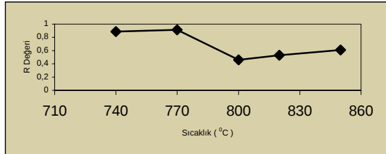
Şekil 4. SAE 1005 sac numunelerinin işlem sıcaklığı - R değeri değişimi
