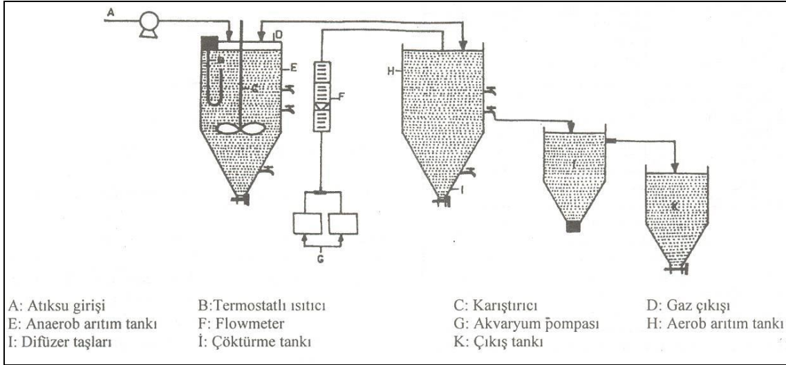
Şekil 4. Araştırmada kullanılan biyolojik arıtmaya ilgili pilot tesis düzeneği.
