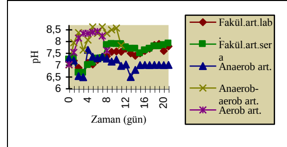
Şekil 5. pH 'nın zamana göre değişimi
