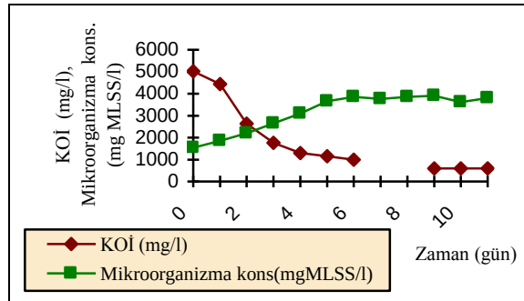
Şekil 7. Organik madde tüketimi ile mikroorganizma büyümesi arasındaki bağıntının grafik olarak gösterilmesi.
