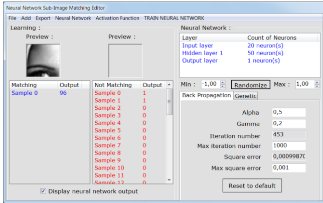
Şekil 8: Yapay sinir ağı eğitim arayüzü ana formu.
