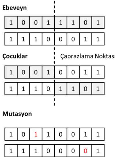
Şekil 4: Çaprazlama ve mutasyon örnekleri.
