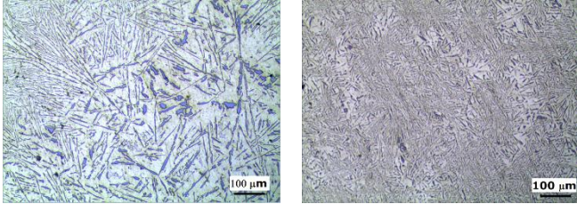
Şekil 4: Al12Si alaşımına ait mikroyapı görüntüleri. (a) Modifiyesiz, (b) Modifiyeli
