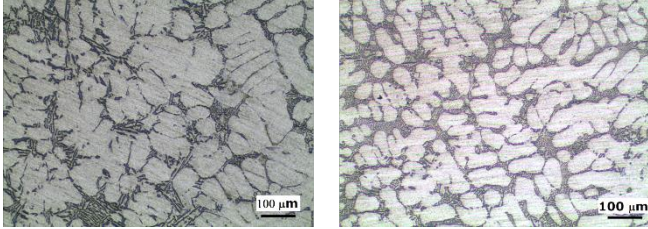
Şekil 3: Al7Si alaşımına ait mikroyapı görüntüleri (a) Modifiyesiz, (b) Modifiyeli
