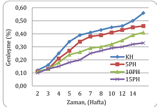
Şekil 3: Harç numunelerinin MgSO 4 çözeltisindeki genleşmeleri.
