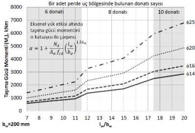
Şekil A1: 200 mm kalınlığa sahip perdelerin taşıma gücü moment abağı.
