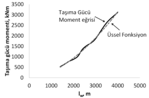
(b): l_w 'nin taşıma gücü momentine etkisi.
