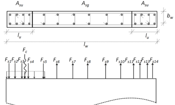
(a): Gerçek perde kesiti ve iç kuvvet dağılımı.
