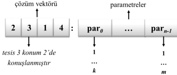
Şekil 2: Kromozom yapısı.
