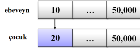
Şekil 4: Mutasyon işlemi.
