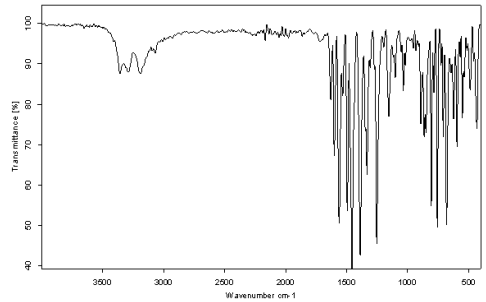
EK 6: CuasalClabt kompleksinin IR spektrumu.
