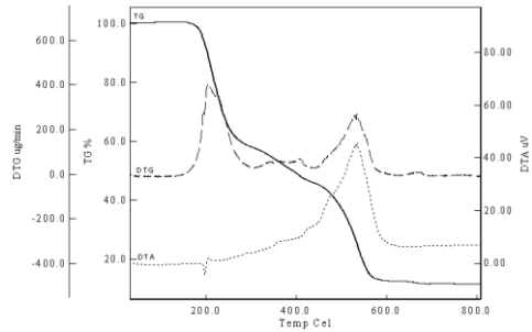
Ek 8: Cuasalabt kompleksinin TG/DTA spektrumu.
