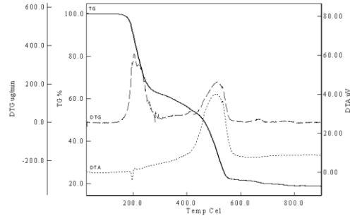
Ek 9: CuasalClabt kompleksinin TG/DTA spektrumu.
