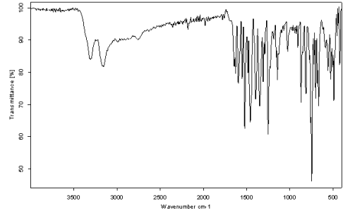
Ek 5: Cuasalabt kompleksinin IR spektrumu.
