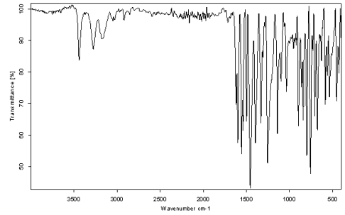
Ek 7: CuasalMeabt kompleksinin IR spektrumu.
