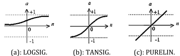
Şekil 1: Transfer fonksiyonları.
