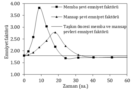
Şekil 7: Memba ve mansap şevleri emniyet faktörlerinin, tren yükü olmaksızın, taşkın anında zamana bağlı değişimi.
