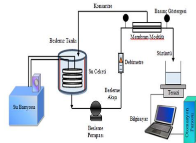
Şekil 1: Sürekli işletimli çapraz akış membran filtrasyonu [19].
