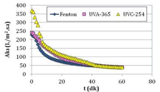
Şekil 4: Konsantrelerin bütünleşik İOP/batık UF hibrit prosesi ile arıtımında UF membranlara ait süzöntü akı değerleri.
