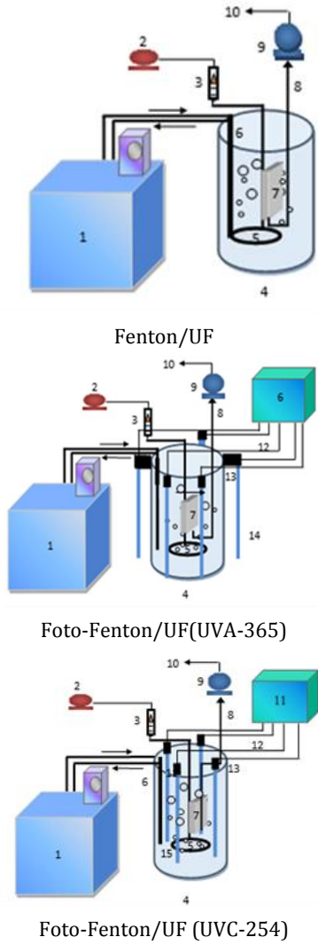
1: Su banyosu, 2: Hava pompası, 3: Debi m, 4: İOP/UF hibrit reaktörü, 5: Difüzör, 6: Online sıcaklık ölçer, 7: Batık UF membran, 8: UF süzünü hattı, 9: Peristaltik pompa, 10: UF süzünü, 11: Güç paneli, 12: Elektrik hattı, 13: Lamba bağlantısı, 14: UVA lambası, 15: Kuvarz camla kaplı UVC lambası.
