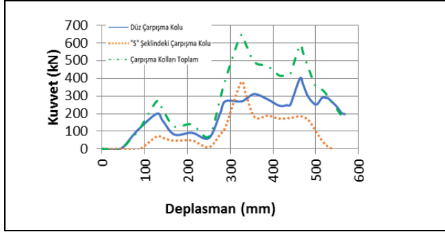
Şekil 12. SÇB için düz ve 'S' şeklindeki çarpışma kollarından yolcu kabinine iletilen kuvvetin deplasmana bağlı değişimi.
