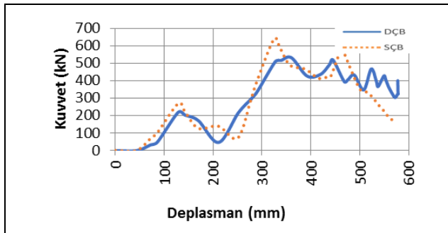
Şekil 13. DÇB ve SÇB için yolcu kabinine iletilen kuvvet ve aracın çarpışma elemanlarının toplam deplasmanı (aracın ezilmesi).
