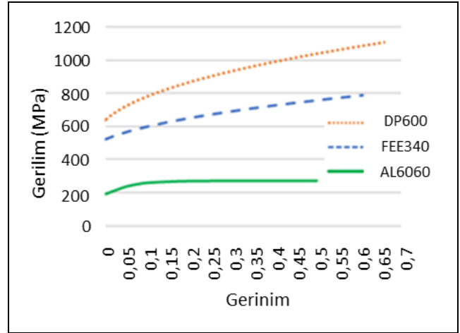
Şekil 8. FEE340 ve DP600 çelik ve AL 6060 alüminyum malzemelerin plastik şekil değiştirme eğrileri.
