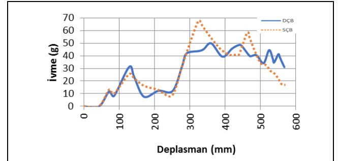
Şekil 15. DÇB ve SÇB için yolcu kabini yavaşlama ivmesinin aracın çarpışma elemanlarının toplam deplasmanı (aracın ezilmesi) ile değişimi.
