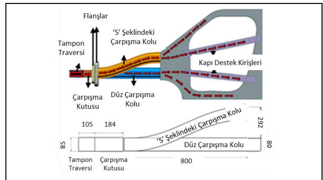
Şekil 6. 'S' şeklindeki çarpışma kolu ile güçlendirilmiş ön çarpışma bölgesinin (SÇB) yük yolu dağılımı ve iki boyutlu ölçülendirmesi.
