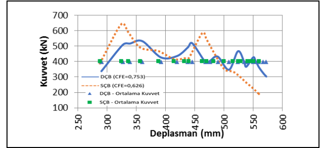
Şekil 14. DÇB ve SÇB için, çarpışma kollarının kuvvet-deplasman eğrisi ve ortalama kuvvet (parantez içindekiler çarpışma kollarının CFE değerlerini ve doğrusal çizgiler ortalama kuvveti göstermektedir).
