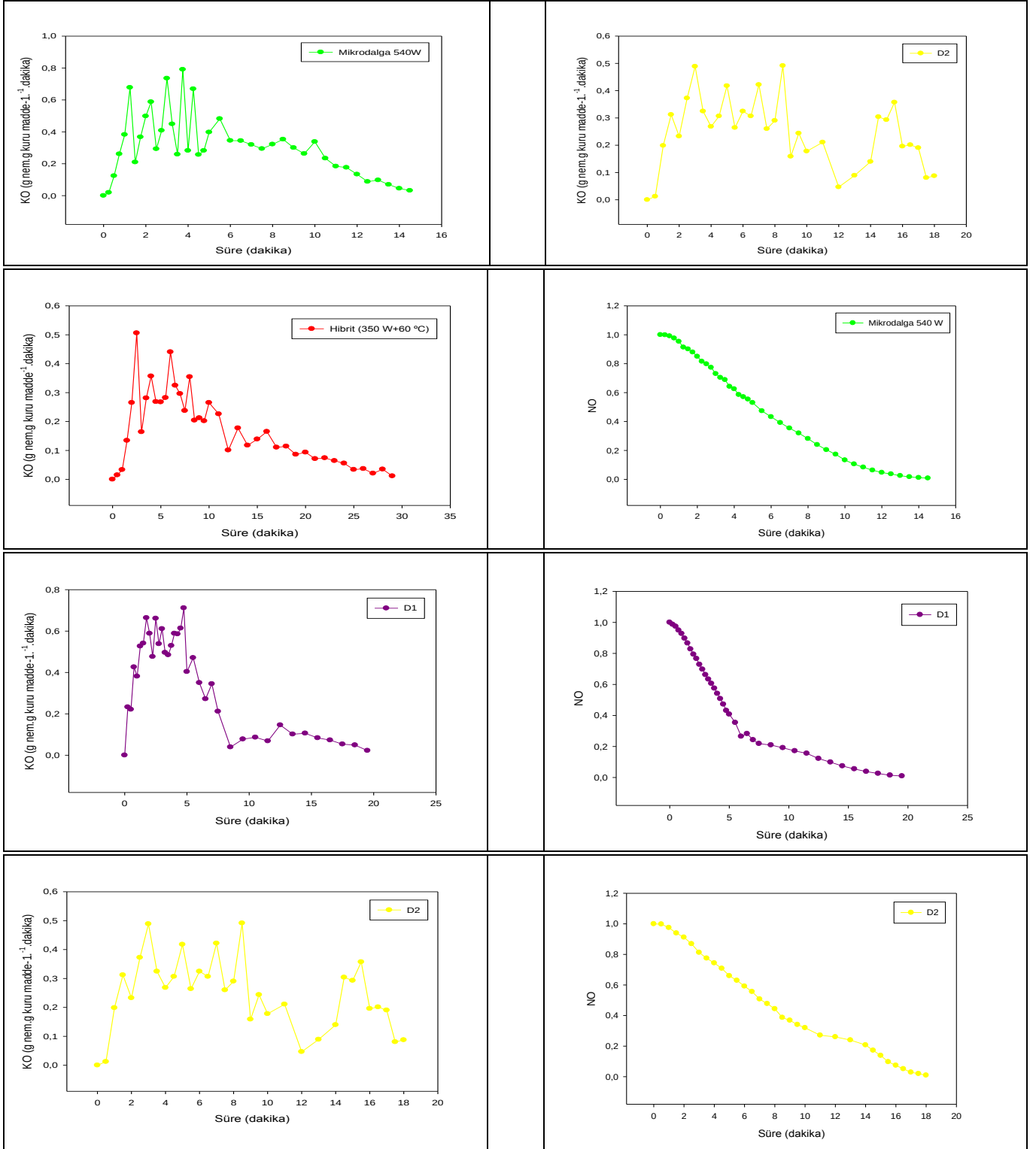
Şekil 1. Göksulu armut örneklerinin kuruma kinetiği.
