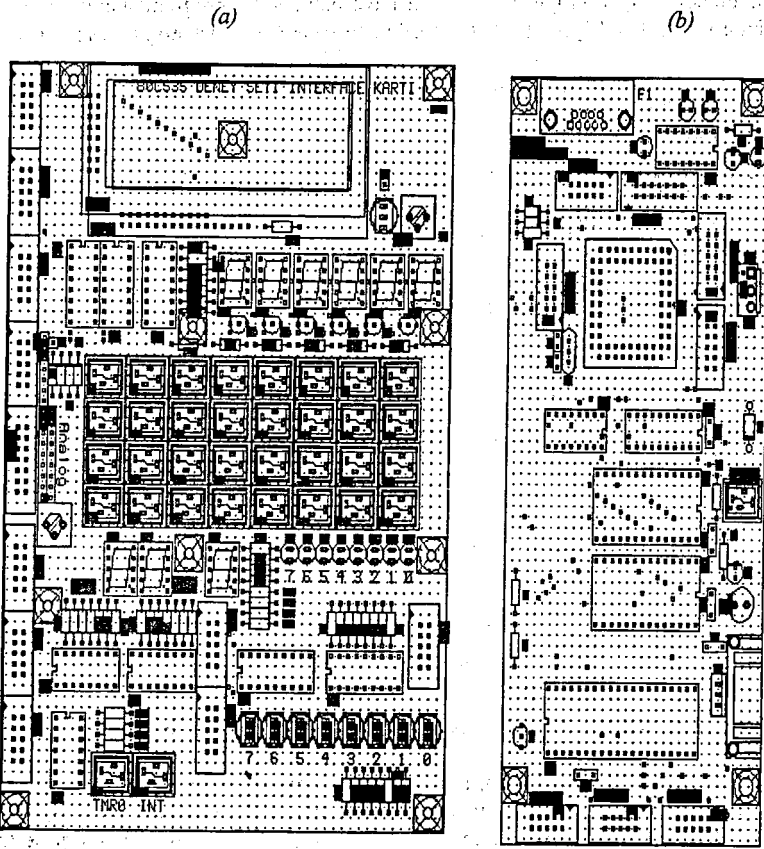
Şekil 1. Mikroişlemcili sistem geliştirme setinin eleman yerleştirme tarafından görünüşü (a)- I/O interface kartı, (b)- CPU kartı.
