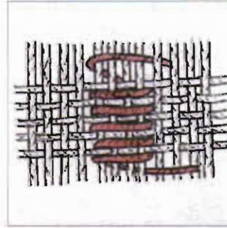
Desen 19. Desen ipliğinin çözgülere dikey sarılması.
