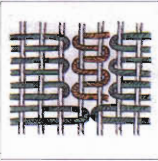
Desen 4. İlikli kilim dokuma tekniği.
