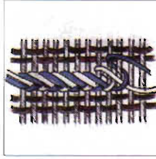
Desen 25. İki değişik renkli desen ipliğinin çözgölere aynı zamanda paralel sarılması.
