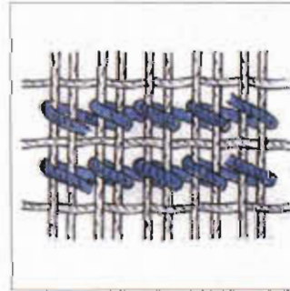
Desen 22. Desen ipliğinin çözgülere içten dışa sarılması.
