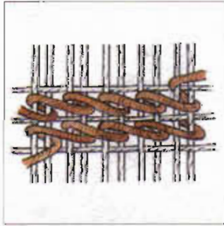
Desen 18. Desen ipliğinin arasından normal atkı geçirilmesi.
