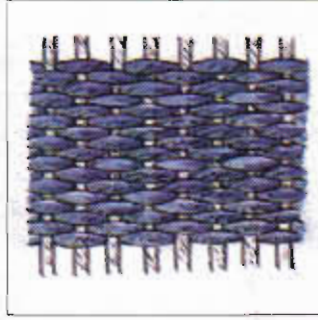
Desen 2. Atkı yüzü dokuma.
