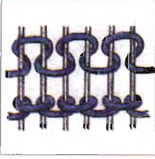
Desen 24. Desen ipliğinin çözümlere üstten ve arkadan sarılması.
