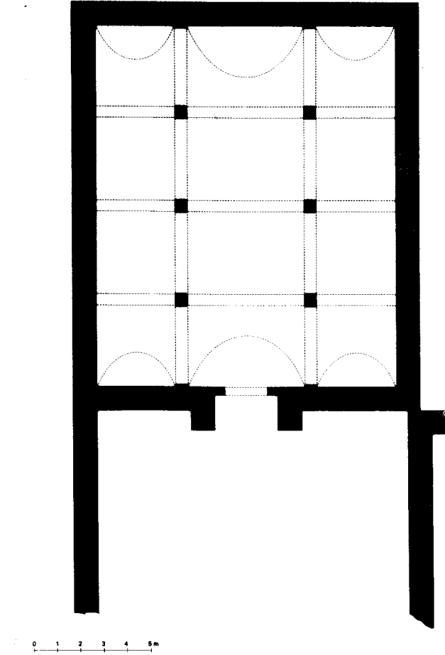
Şek.2- Elikesik Han Planı.
