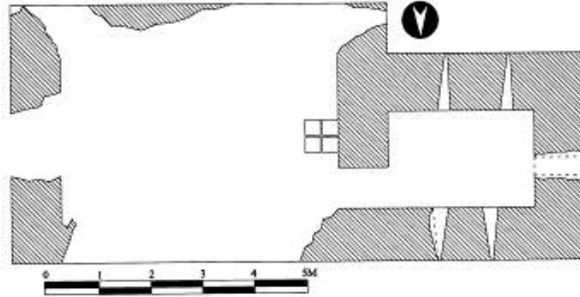
Şek.2- Alanya Çıplaklı Mahallesi'ndeki Selçuklu Köşkü (üst kat) (Rölöve-Çizim: Aytekin Yavaş)
