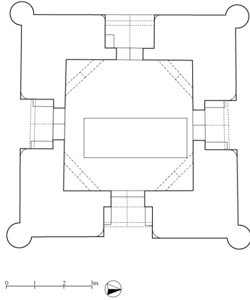
Şek. 1- Jambul, Ayşe Bibi Türbesi, plan
