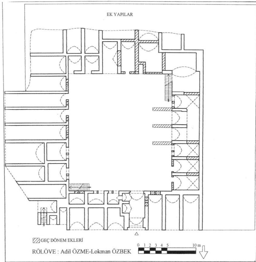
Şek.1- Barutçu Hanı, alt kat rölöve planı
