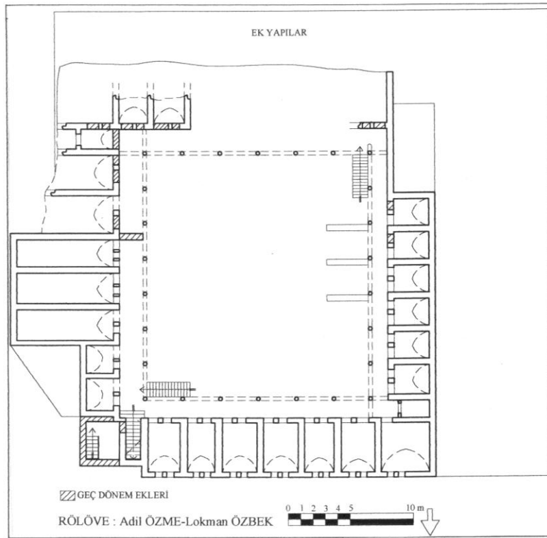
Şek.2- Barutçu Hanı, üst kat rölöve planı
