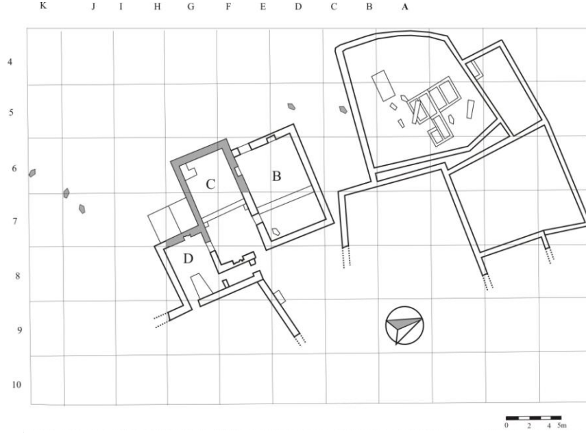
Şek.5- Menteşe Mezarlığı. Plan. (2006 yılı bulguları, E. Daş'ın çizimi üzerine B. Sağıt tarafından işlenmiştir).
