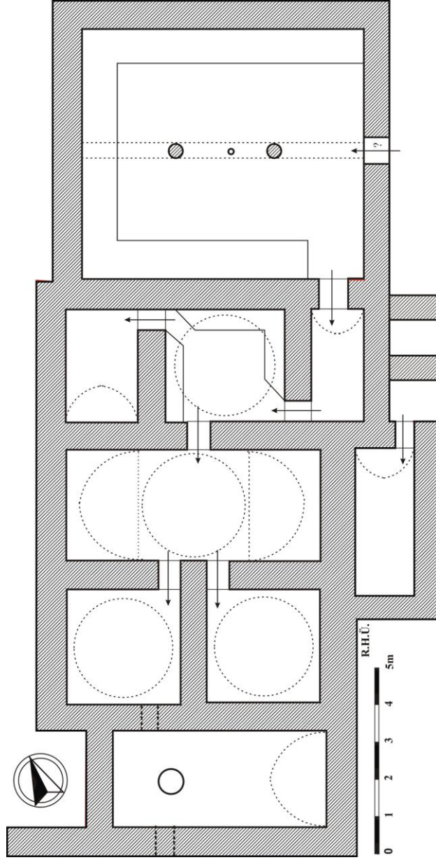
Şekil 3-Seymenlik Hamamı. Restitüsyon Planı. (Ş Çakmak'ın rölöve planı esas alınmıştır.)
