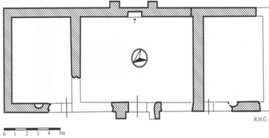
Şek. 4- Lokman zaviyesi plan taslağı.
