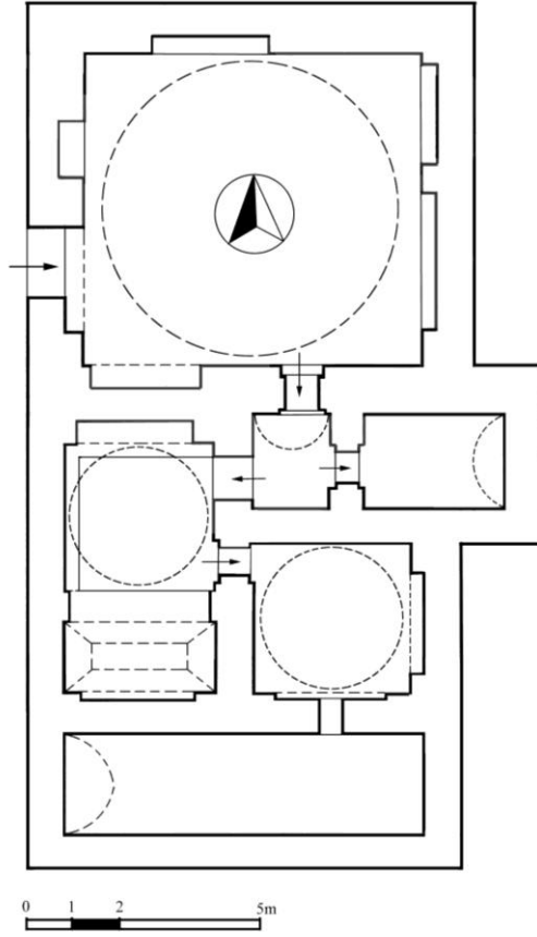
Şekil 2- Manisa Saray Hamamı. Restitüsyon denemesi.
