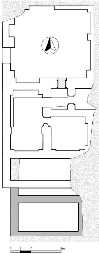
Şekil 1- Manisa Saray Hamamı. Plan.
