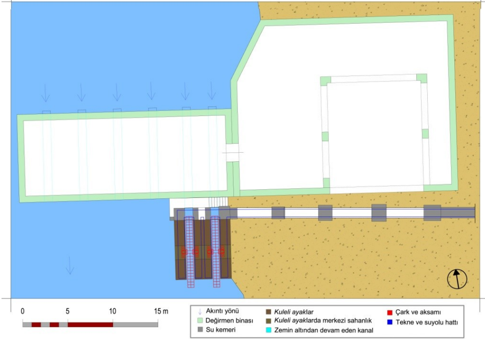
Plan.4- 'Alvân Su Kemerı restitüsyon planı (II). (E. Özbay)
