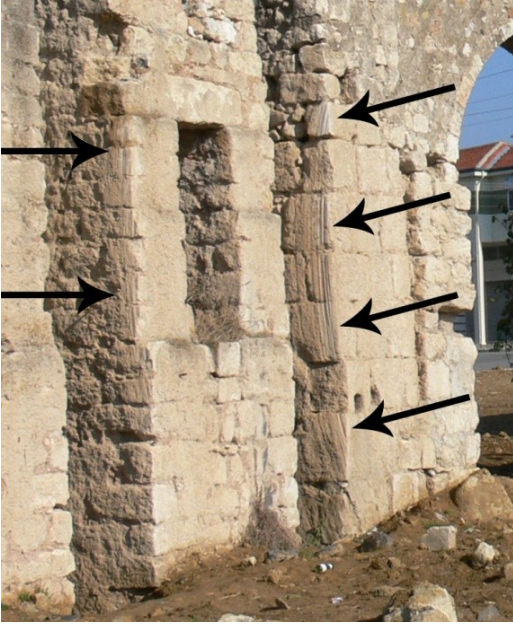
Res.16- ‘Alvân Su Kemer; başlangıç bölümü; kemer gözlerinde sürtünme izleri. (Güneyden)
