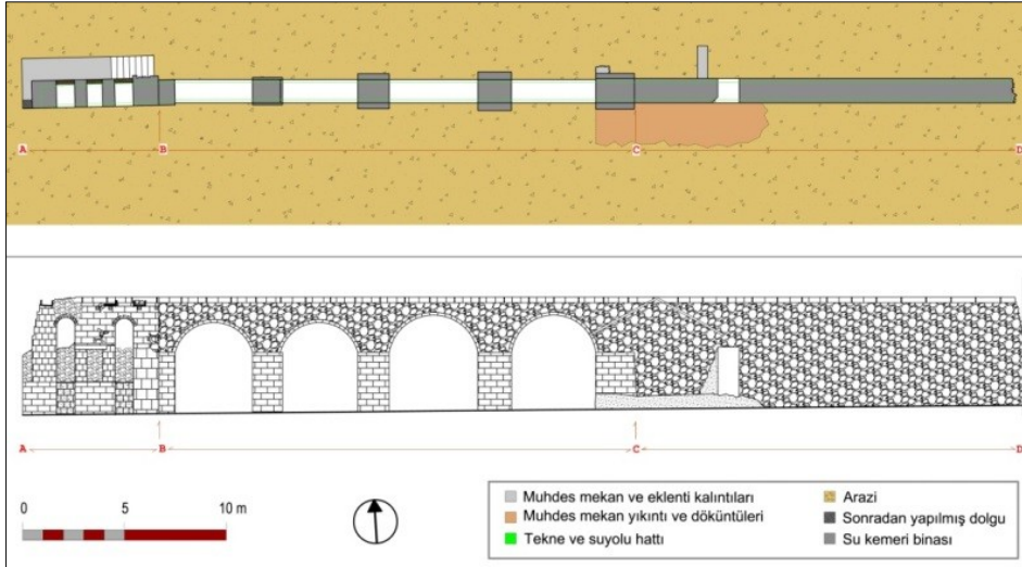
Plan.1- ‘Alvân Su Kemer Kalıntısı vaziyet planı. (E.Özbay)
