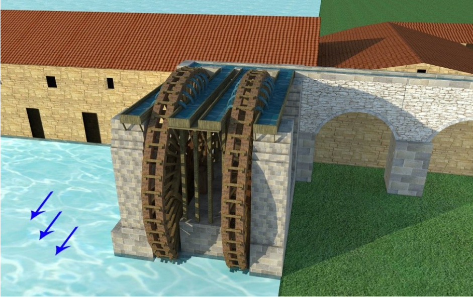
Şek.7- ‘Alvân Naurası, Su Kemerı ve Değirmeni rekonstrüksiyon modeli. (V) (E.Özbay)
