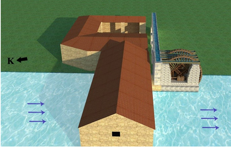
Şek.5- ‘Alvân Nurası, Su Kemerı ve Değirmeni rekonstrüksiyon modeli. (III) (E.Özbay)
