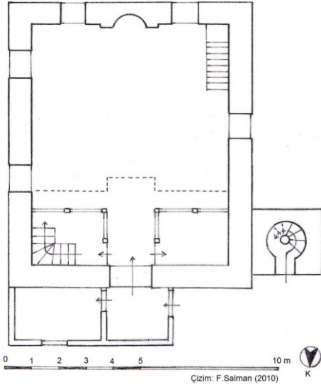
Çizim 2- Ilıpınar Köyü Hacı Serdar Camii'nin Planı
