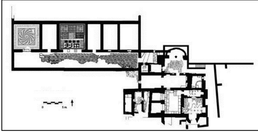
Resim 1: Antandros’da açığa çıkarılan Geç Antik villanın planı ( Polat vd. 2008, s:470. plan:1)
