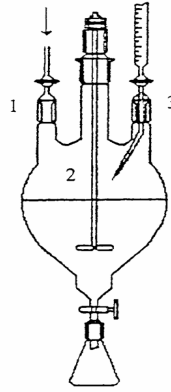
Şekil 1. Fraksiyonlaştırma düzeneği: (1) Azot gazı girişi (2) Mekanik karıştırıcı (3) Çöktürücü girişi.
