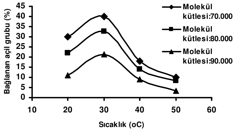
Şekil 3. PS yapısına bağlanan açıl grubu miktarı ile sıcaklık arasındaki ilişki.
