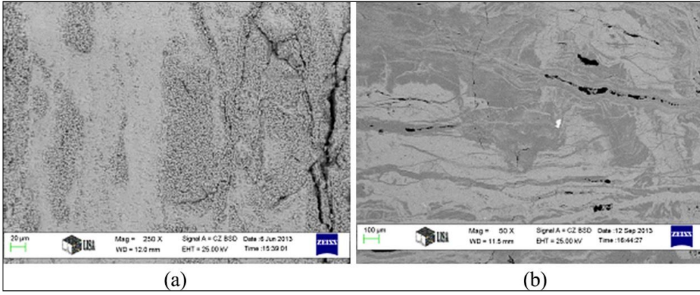
Foto 6- El Markab Kalesinde bir temrenin SEM görüntüsü (Török vd., Fig.6)
