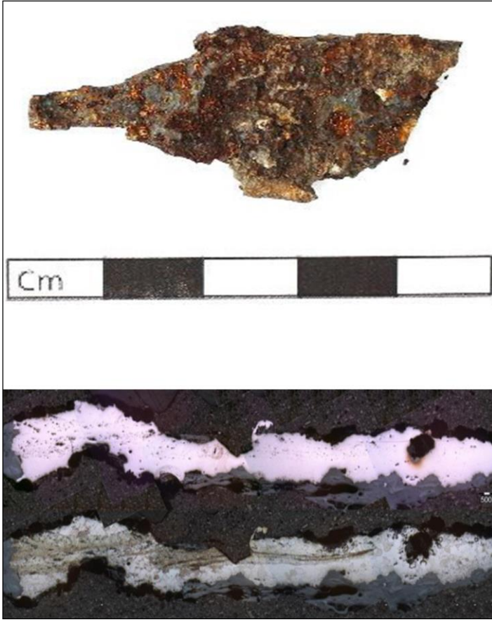
Foto 16- Kinet Höyükte bulunmuş KH-06 numaralı temren ve dağlanma öncesi-sonrası içyapı görüntüsü (Güder, s.134.)
