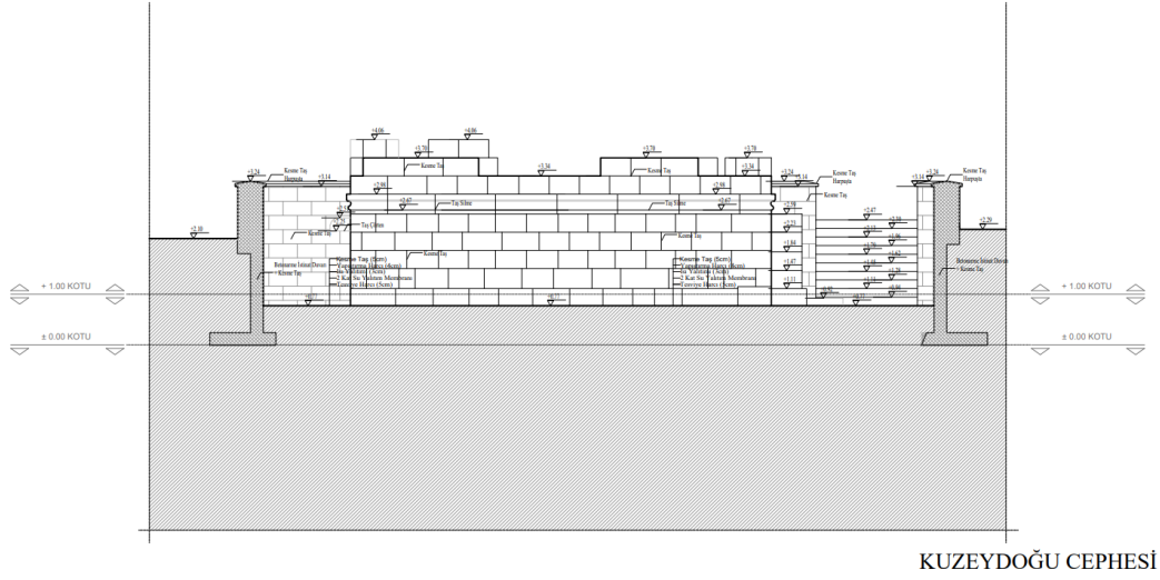
Çizim 3: Kuzeydoğu Cephesi
