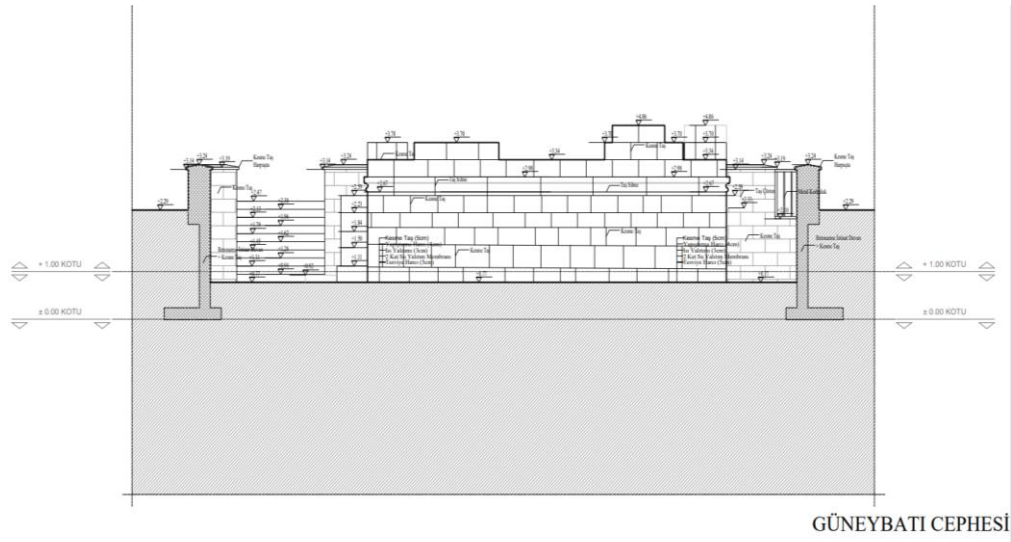
Çizim 5: Güneybatı Cephesi
