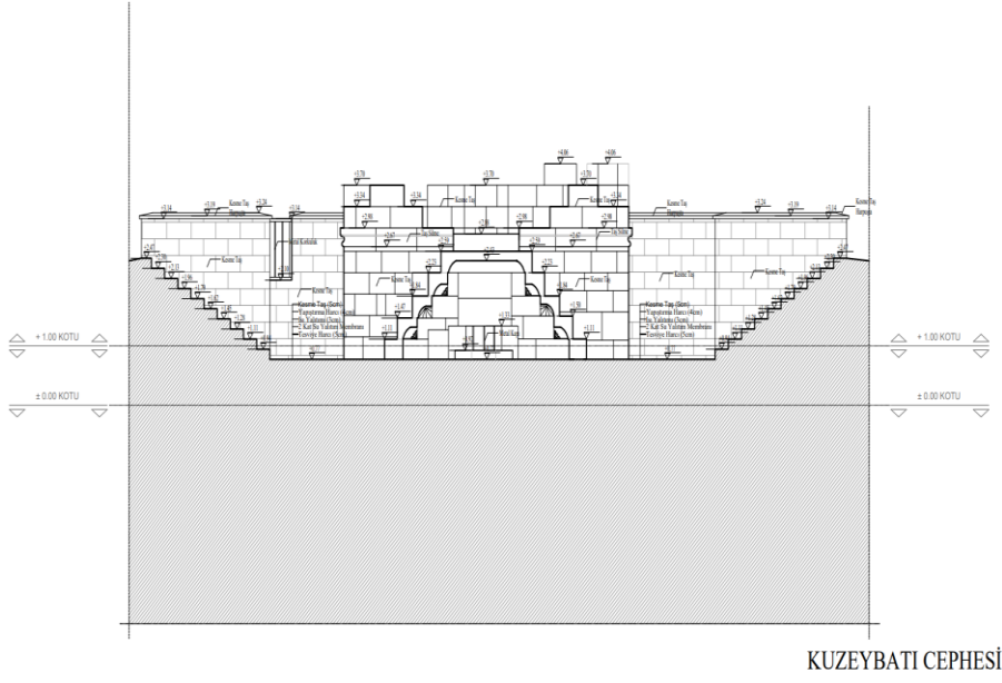
Çizim 2: Kuzeybatı Cephesi
