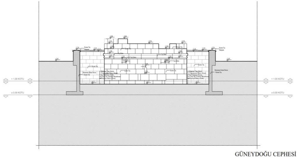
Çizim 4: Güneydoğu Cephesi
