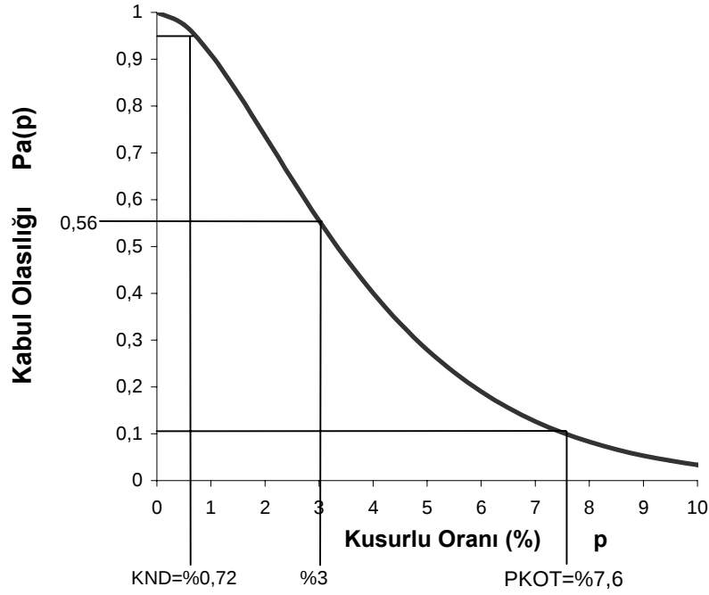
Şekil 1. n=50 , c=1 Değerleri ile Verilen B Tipi Tekli Örneklem Planının İK Eğrisi.
