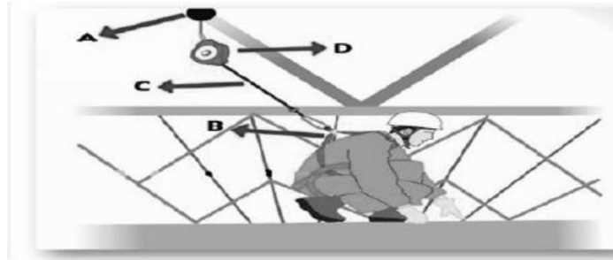
Ankraj Noktası, B-Paraşüt Tipi Emniyet Kemer, C-İçeri Çekilebilir Bağlantı Elemanı, D- Geri Sarmalı Düşme Durdurma Sistemi
