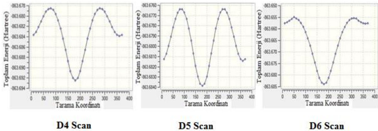
Şekil 2. 2-[(4-Hidroksifenil)diazenil]benzen-1,3,5-triol molekülü için HF/3-21G metoduyla hesaplanan D1-6 dihedral açılarının dönme enerji eğrileri
