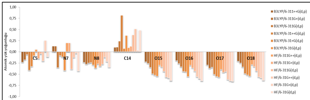
Şekil 4. 2-[(4-Hidroksifenil)diazenil]benzen-1,3,5-triol molekülünün B3LYP ve HF metodlarının farklı temel setlerine göre atomik yük yoğunluklarındaki değişimi
