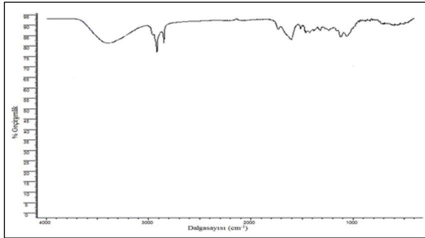
Şekil 6. 2-[(4-Hidroksifenil)diazene]benzen-1,3,5-triol molekülünün FT-IR spektrumu
